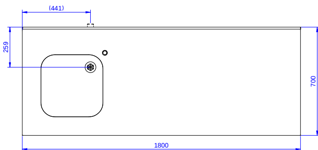
Päältä
